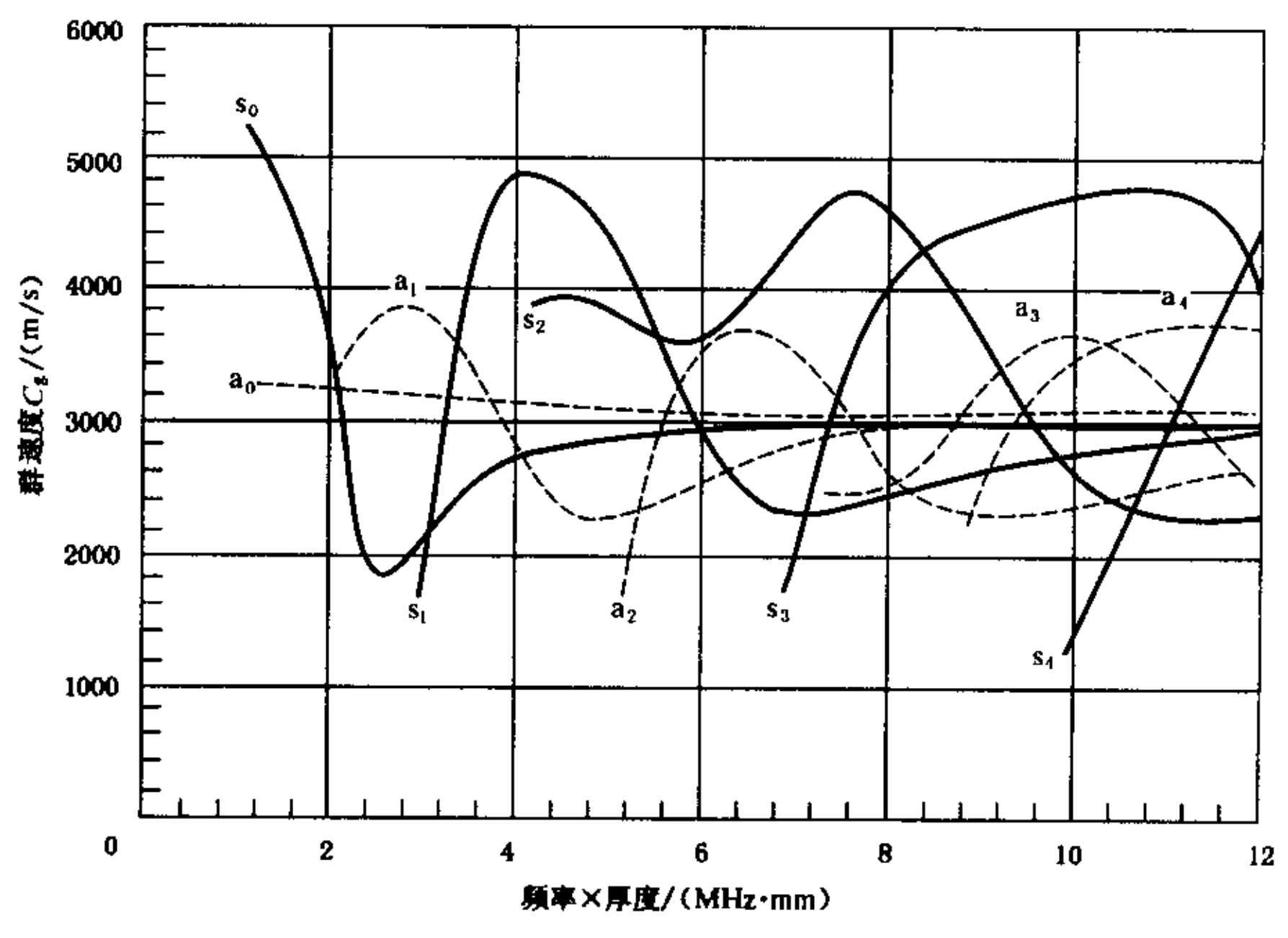
图 F2 Cr17Ni2 材料 Lamb 波群速度曲线
