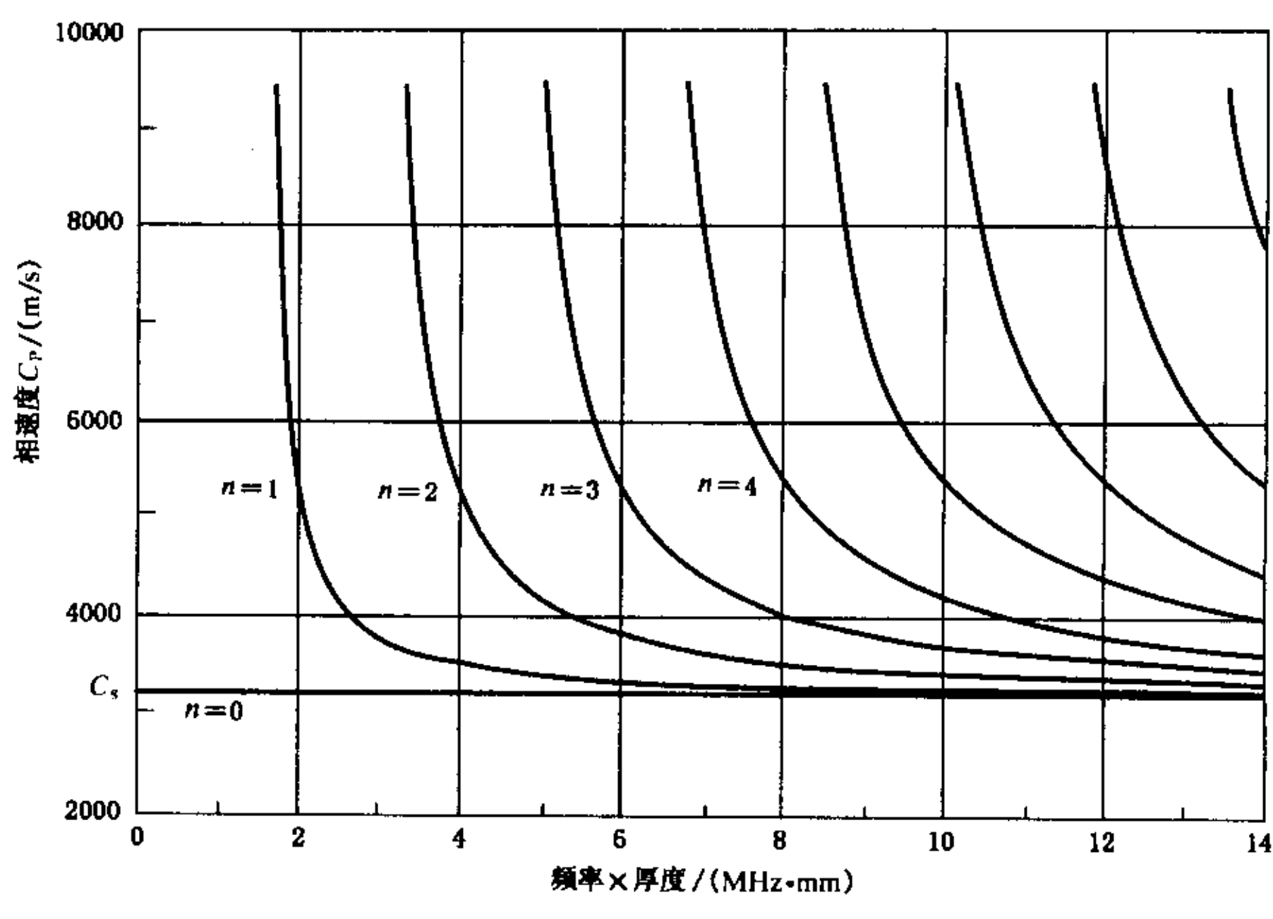
图 B3 406 钢 SH 波相速度曲线
