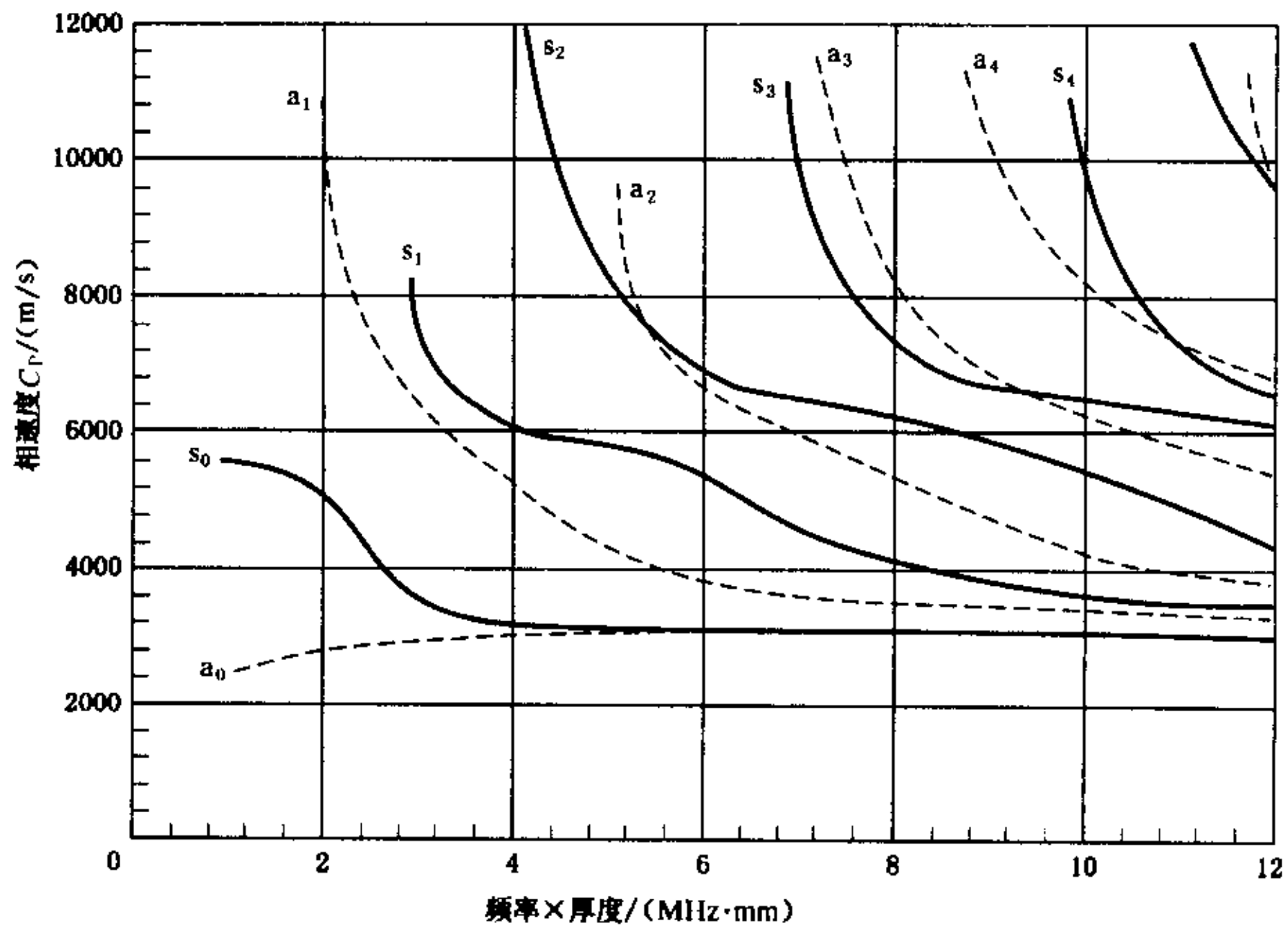
图 F1 Cr17Ni2 材料 Lamb 波相速度曲线
