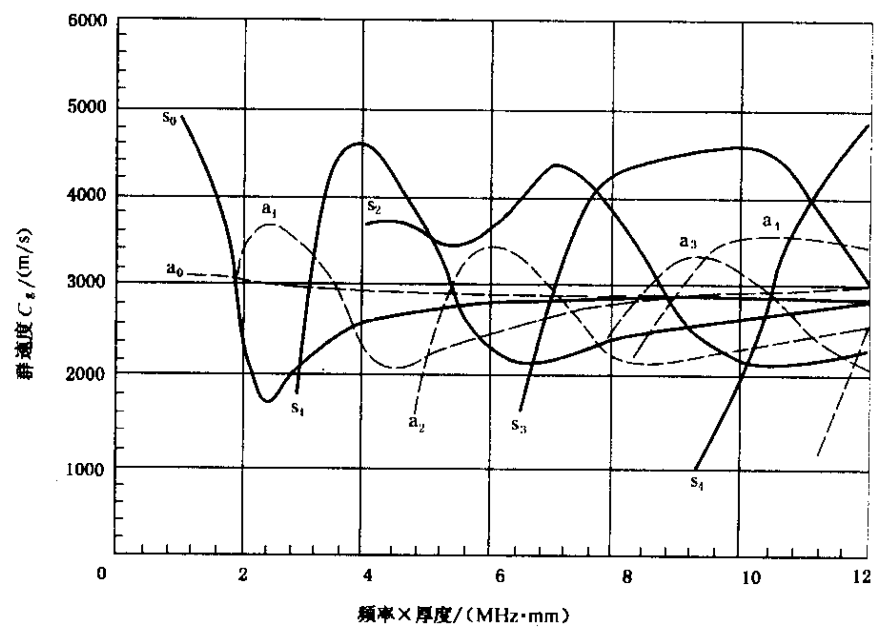
图 G2 GH169 材料 Lamb 波群速度曲线
