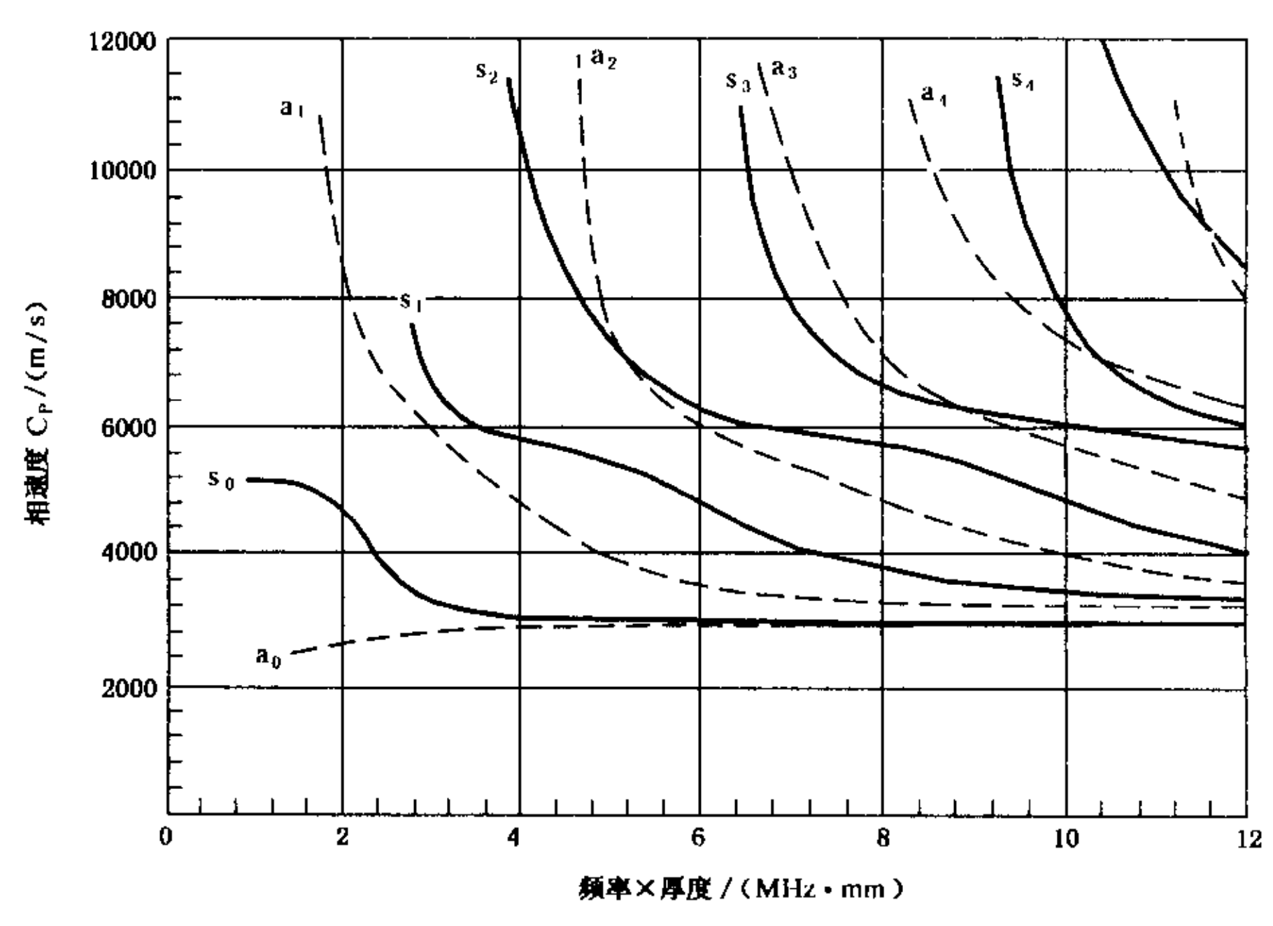
图 J1 TC2 材料 Lamb 波相速度曲线
