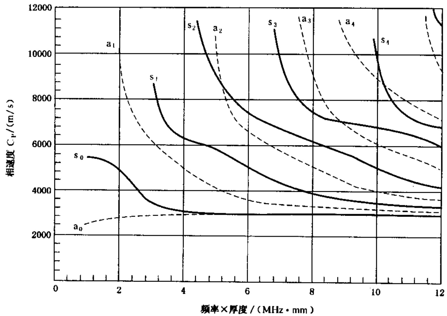
图 L1 5A06 材料 Lamb 波相速度曲线
