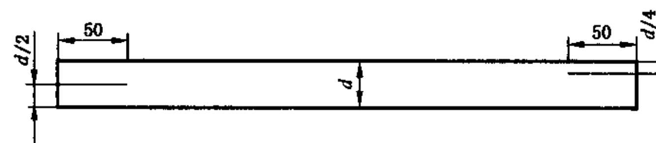
(a) 通孔型对比试样
