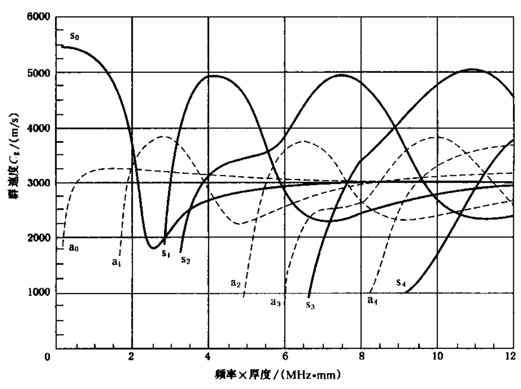
图 C2 低碳钢板 Lamb 波群速度曲线
