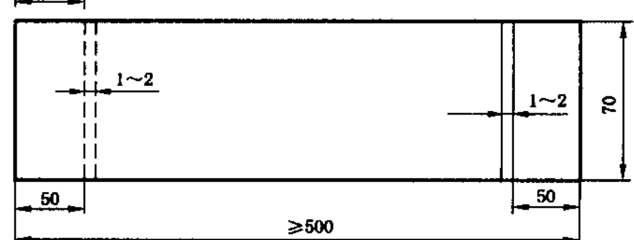
(d) 平底槽型对比试样
