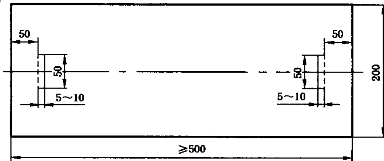
(c) 人工分层(嵌入云母)型对比试样
