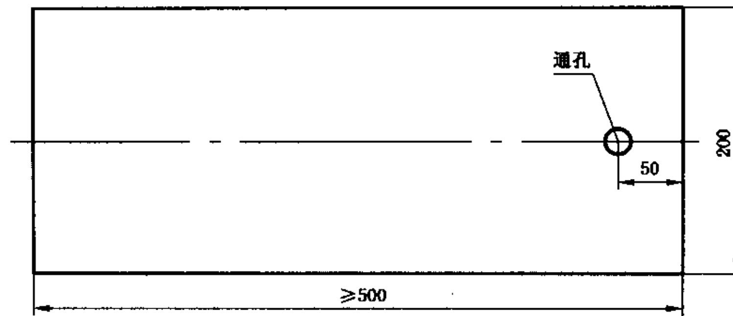
(a) 通孔型对比试样
